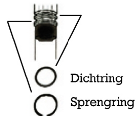
Wasserdurchführungsrohr mit VARIO-fix-System
